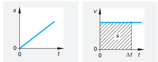
Bild 1: s,t-Diagramm Bild 2: v,t-Diagramm
