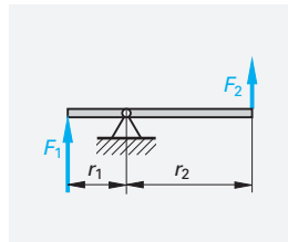
Bild 7: Zweiseitiger ungleicharmiger Hebel
