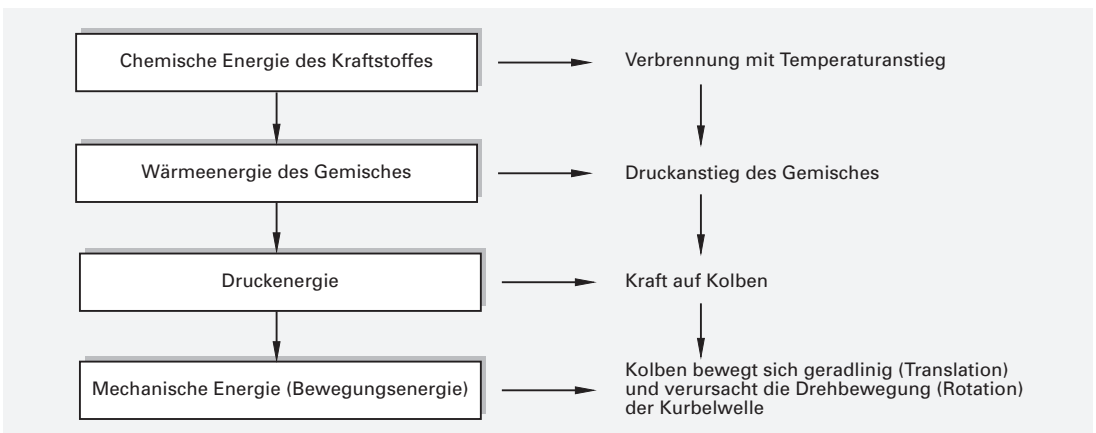
Bild 2: Energieumwandlung in einer Verbrennungskraftmaschine
