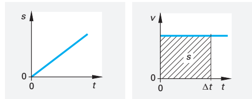
Bild 1: s,t-Diagramm
