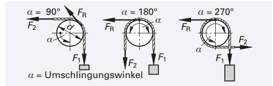
Bild 1: Seilreibung
