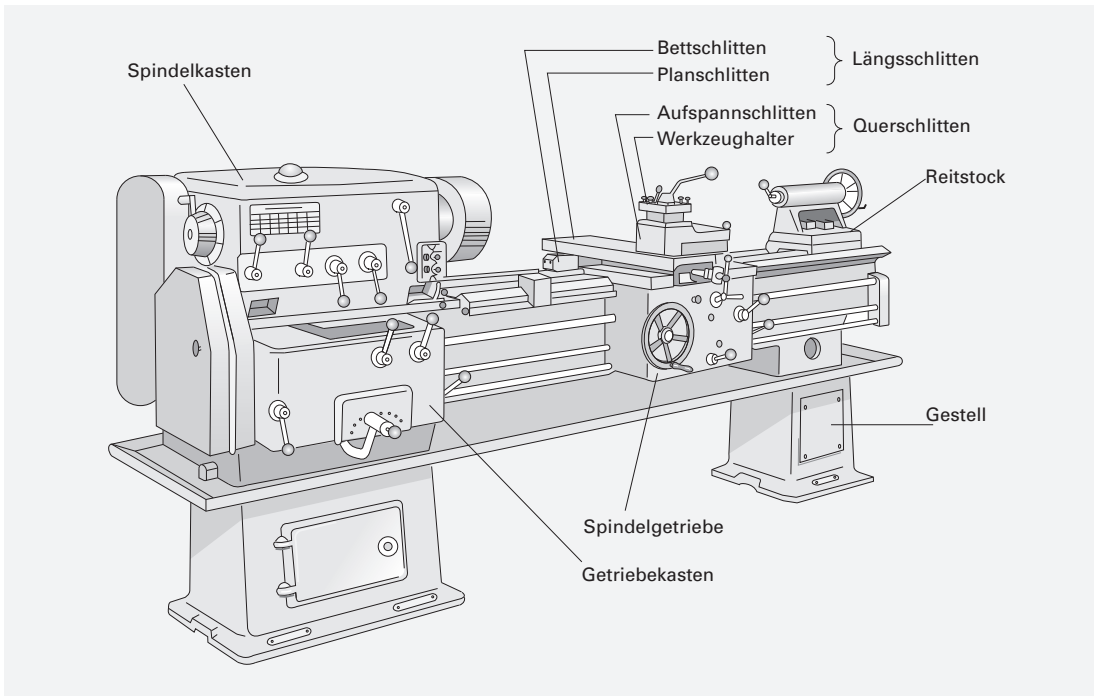
Bild 1: Drehmaschine, aus mehreren Baugruppen zusammengesetzt
