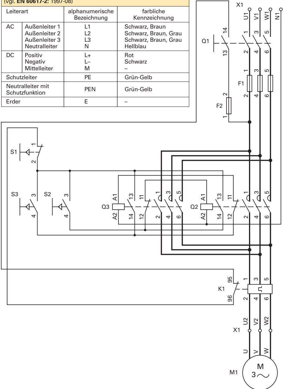
Beispiel 1: Stromlaufplan in zusammenhängender Darstellung Dargestellt ist ein Antriebssystem für 2 Drehrichtungen
