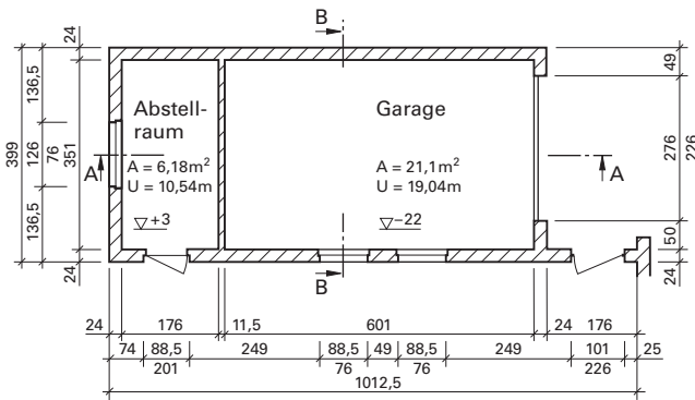
Grundriss
