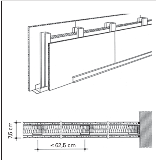
Bild 8.1 Metallständerwand Einfachständerwerk, einfach beplankt
