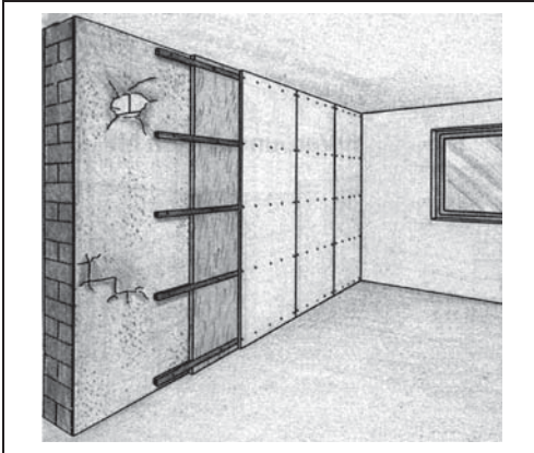
Bild 7.12 Vorsatzschale auf Holzlatten
