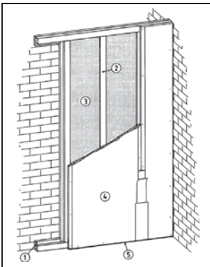
Bild 7.13 Vorsatzschale auf Schwinghölzern
