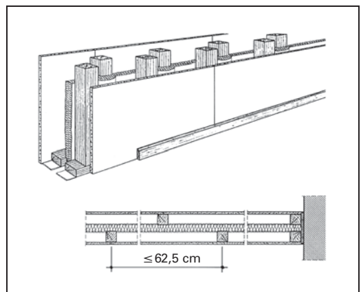
Bild 8.4 Holzständerwand als Doppelständerwerk, zweifach beplankt
