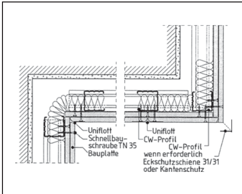
Bild 7.19 Freistehende Vorsatzschalen, doppelt beplankt, Innenecke, Außenecke
