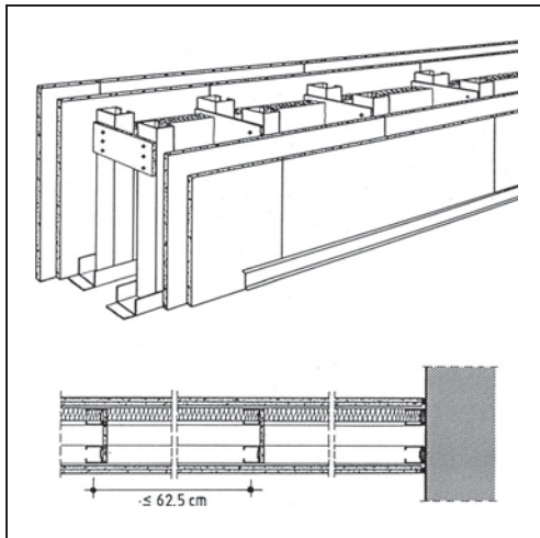
Bild 8.5 Installationswand
