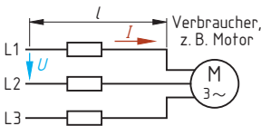
Schaltung bei Drehstrom (3 AC)
