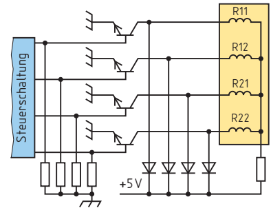
Prinzip einer unipolaren Schrittmotor-Steuerschaltung
