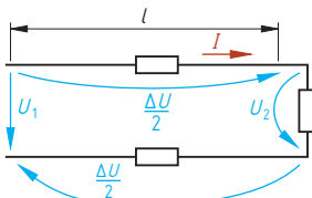
Schaltung bei DC und AC
