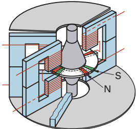
Scheibenmagnet-Schrittmotor
