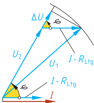
Zeigerbild bei AC
