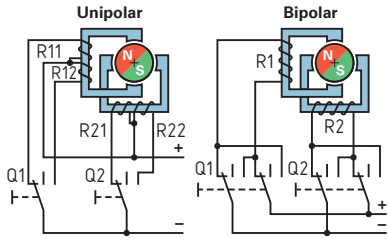
Zweistrang-Schrittmotoren
