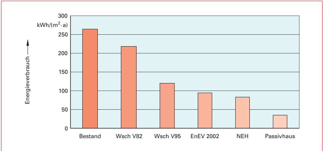
Bild 1.4 Entwicklung des Energieverbrauchs bei einem freistehenden Einfamilienhaus
