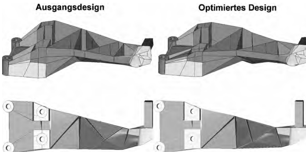
Abb. 8.7 Ausgangsdesign und optimiertes Design des Motorhalters
