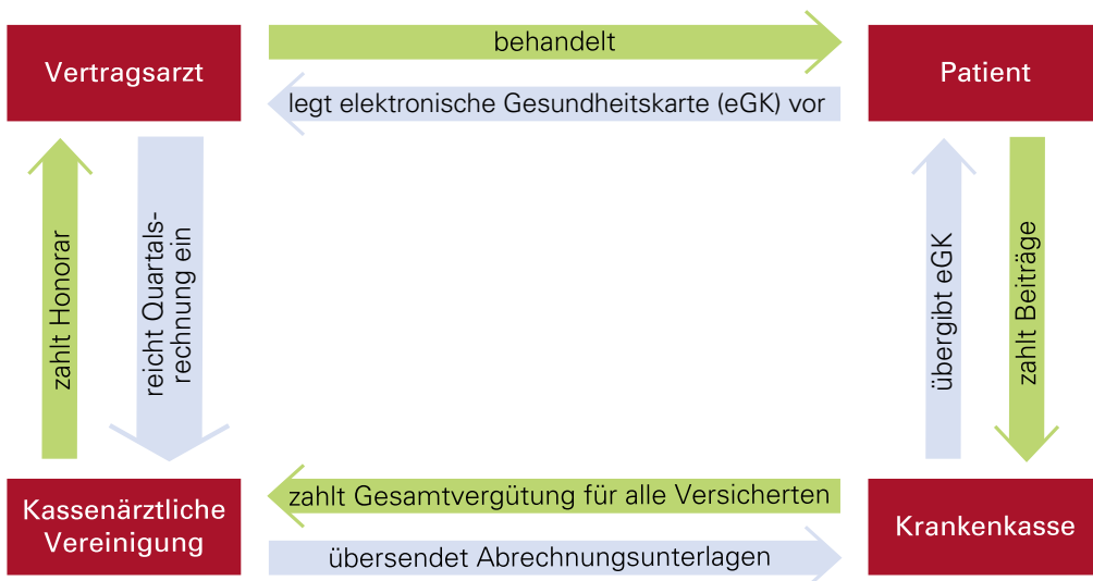
Abb. 1 Kassenärztliches Viereckmodell
