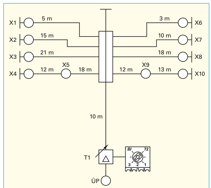
Bild 1: Breitbandkommunikationsanlage
