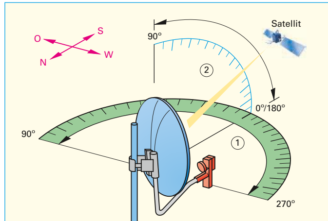
Bild 1: Winkelseinstellung an der Parabolantenne
