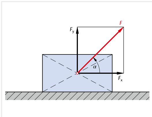
Bild 1: Zerlegung einer Kraft
