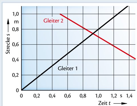
Bild 1: Gemeinsames Zeit-Ort-Diagramm
